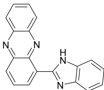
Сполука 1
